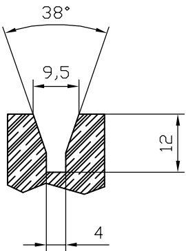
Z 1:1 (Keilrille)
